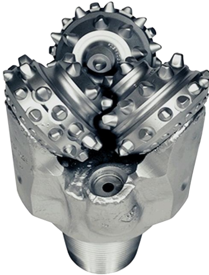
Tungsten Carbide Insert (TCI)
